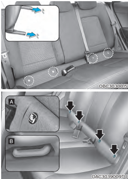
[A] : ISOFIX-kinnituspunkti asukohta tähis, [B] : ISOFIX-kinnituspunkt
