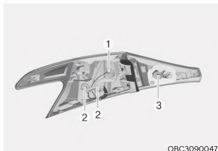
[1] : Suunatuli [2] : Tagatuli/pidurituli [3] : Tagatuli
